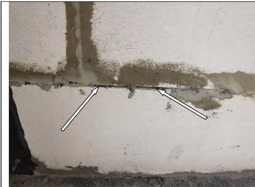
Фото №22. Некачественное выполнение швов кладки из ячеистых бетонных блоков в лоджии.
