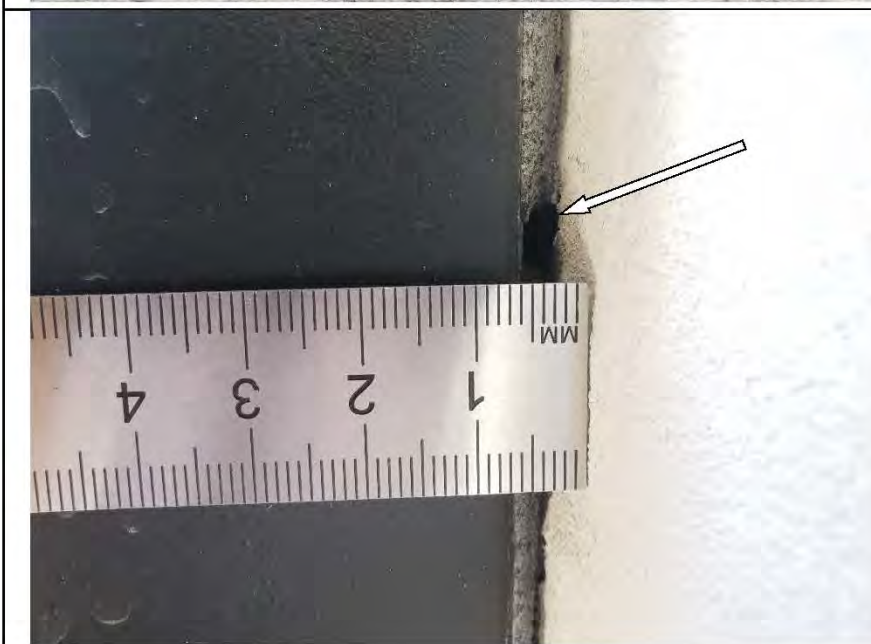
Фото №33. Некачественное выполнение узла примыкания металлического оконного блока к стене на лоджии..
