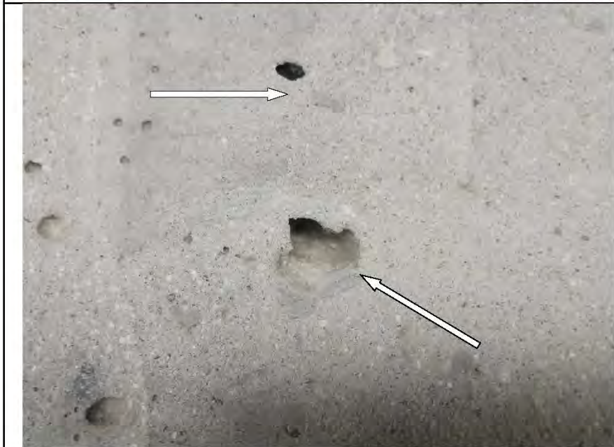
Фото №15. Отсутствие однородности внешнего вида поверхности железобетонного пилона в гостиной.
